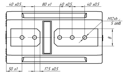
Рис.Г.3 Общий вид трансформатора ТОЛ-10-М-3 на токи от 600 до 2000А. Остальное см. рис.Г.2
