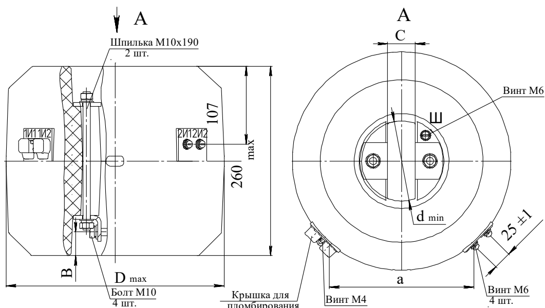
Рисунок Б.1 Общий вид трансформаторов тока ТШЛ-10, ТШЛП-10
