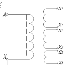
Рисунок Б.4 Принципиальная электрическая схема трансформатора ЗНОЛ.06 4-35
