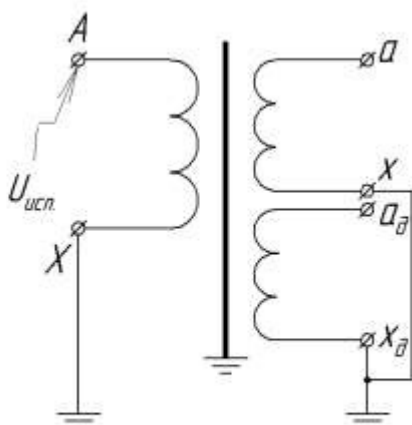
Рисунок Г.3 Схема испытания электрической прочности изоляции первичной обмотки трансформатора приложенным напряжением 1,3 номинального при частоте 50 Гц
