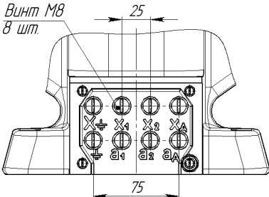
Рисунок Б.2 Клемник для исполнения ЗНОЛ.06 4-35 (остальное – см. рис. Б.1, крышка условно не показана)
