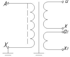
Рисунок Б.3 Принципиальная электрическая схема трансформаторов
