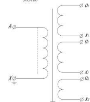
Рисунок А3 Принципиальная электрическая схема для исполнений ЗНОЛ.06.4
