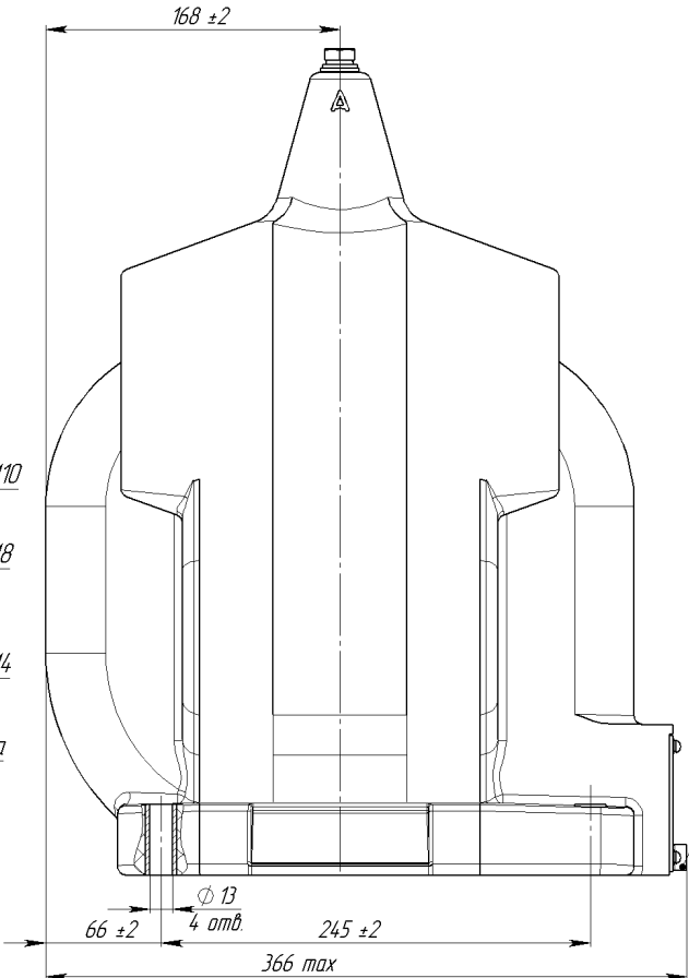
Рисунок Б.2 Клемник для исполнения ЗНОЛ.06 4-35 (остальное – см. рис. Б.1, крышка условно не показана)
