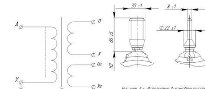
Рисунок А4 Исполнение высоковольтного вывода трансформаторов для такопрободов (остальное см. рисунок А1)
