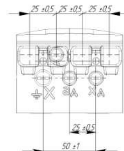
Рисунок А5 Клеммы для четырехобмоточных трансформаторов (остальное см. рисунок А1)
