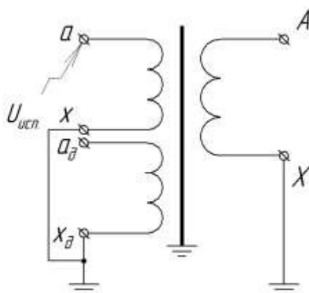
Рисунок Г.2 Схема испытания электрической прочности изоляции первичной обмотки трансформатора индуктированным напряжением частотой 400 Гц
