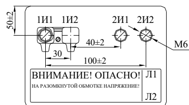
Рисунок Б.1 Трансформаторы тока ТШЛ-20-1
