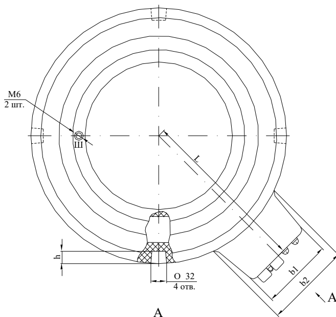
Рисунок Б.2 Трансформаторы тока ТШЛ- 20-1-3 (остальное см. рисунок Б.1)
